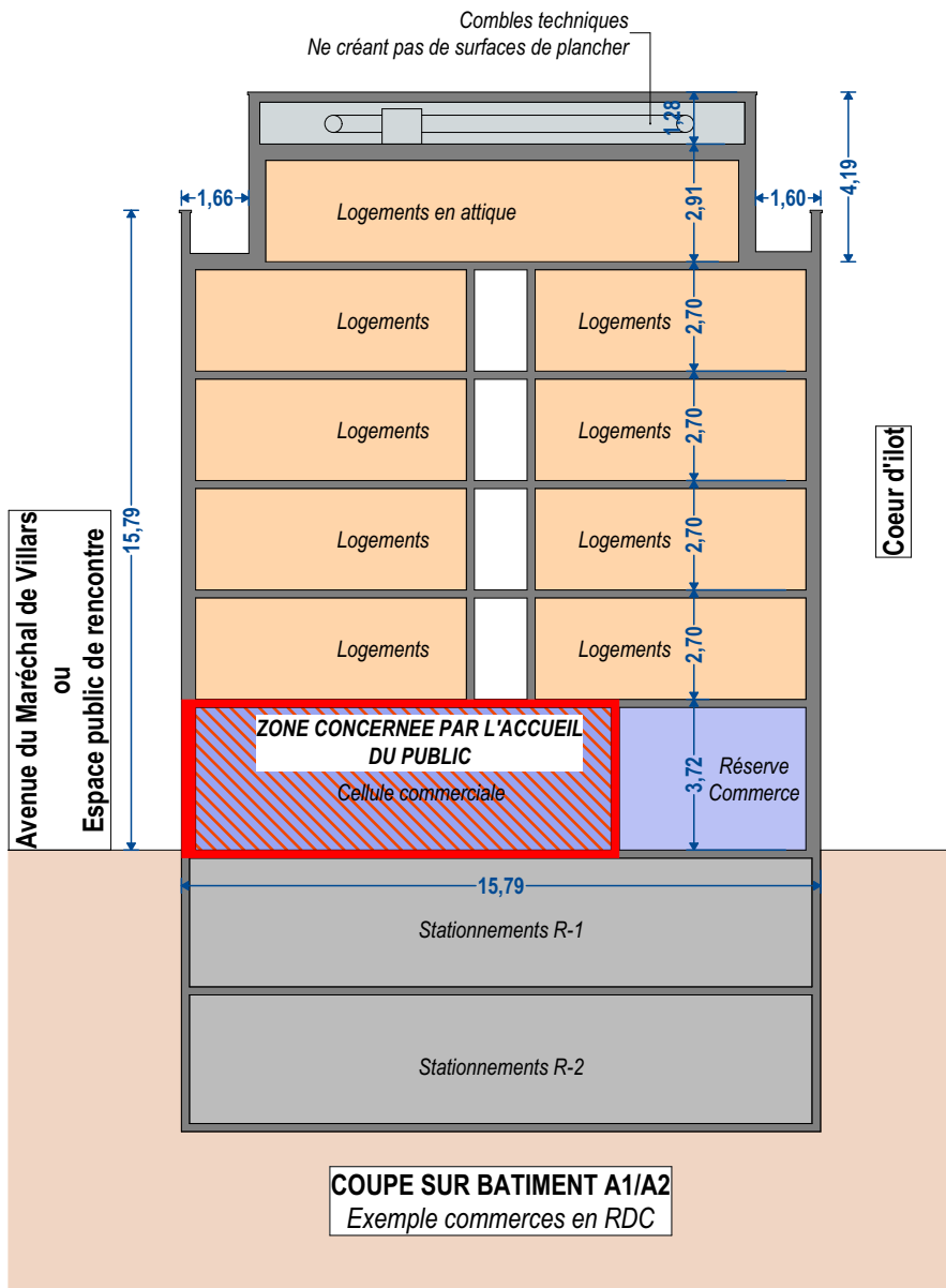
COUPE 1
