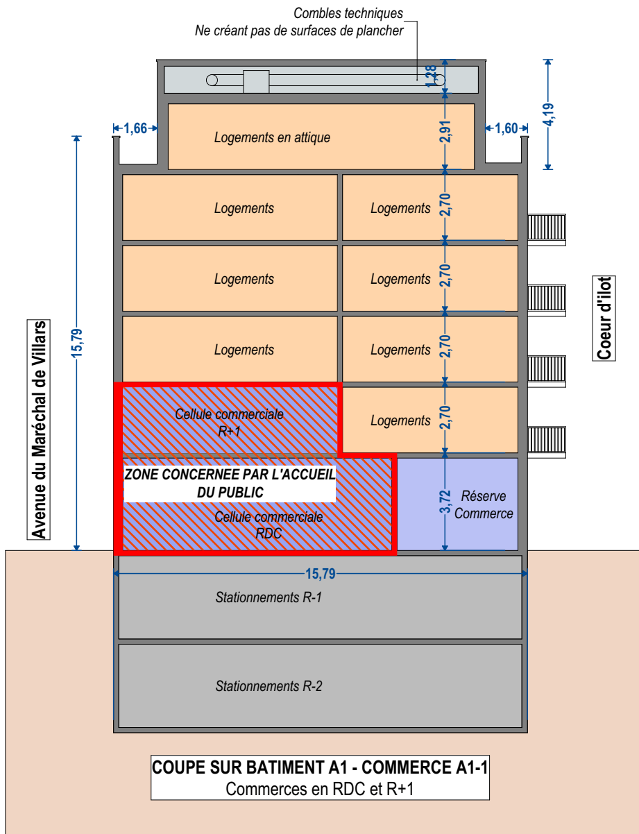
COUPE 2
