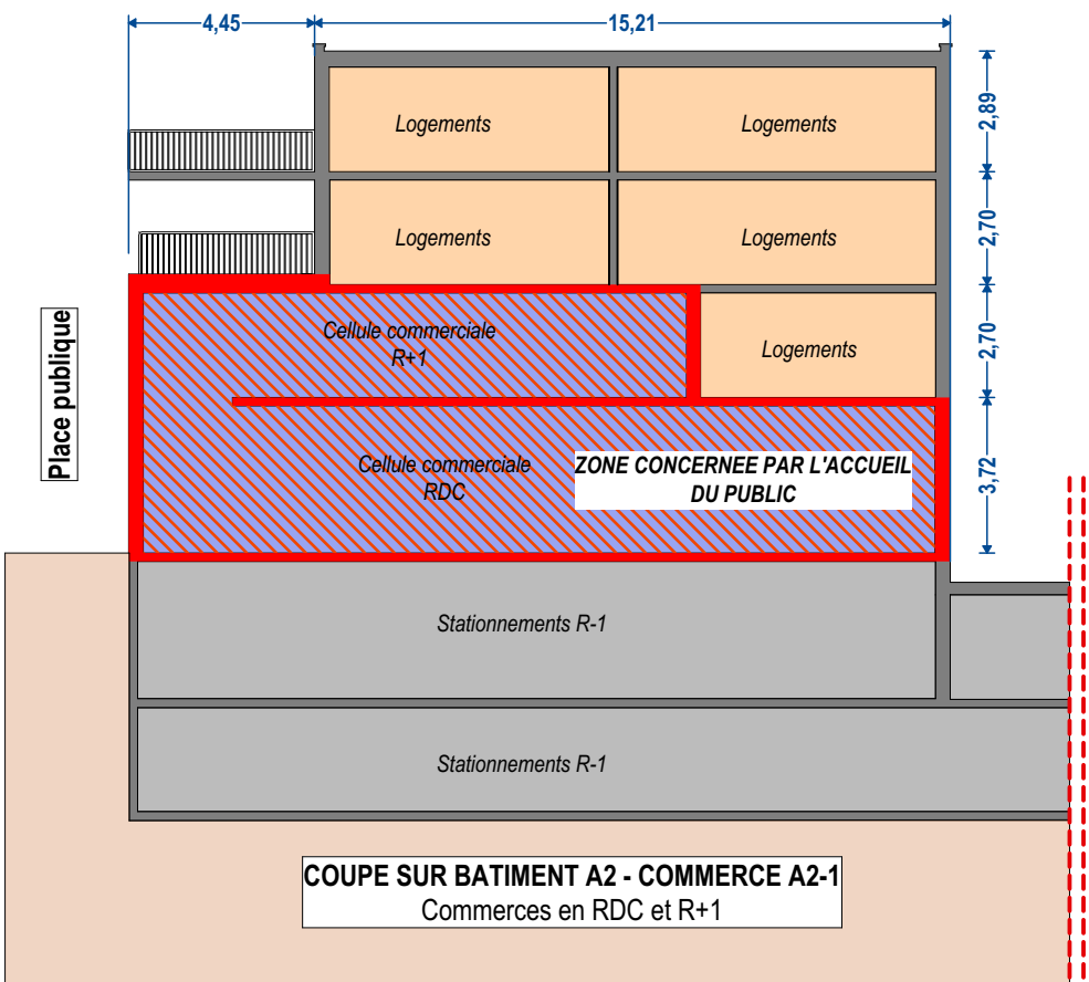
COUPE 3
