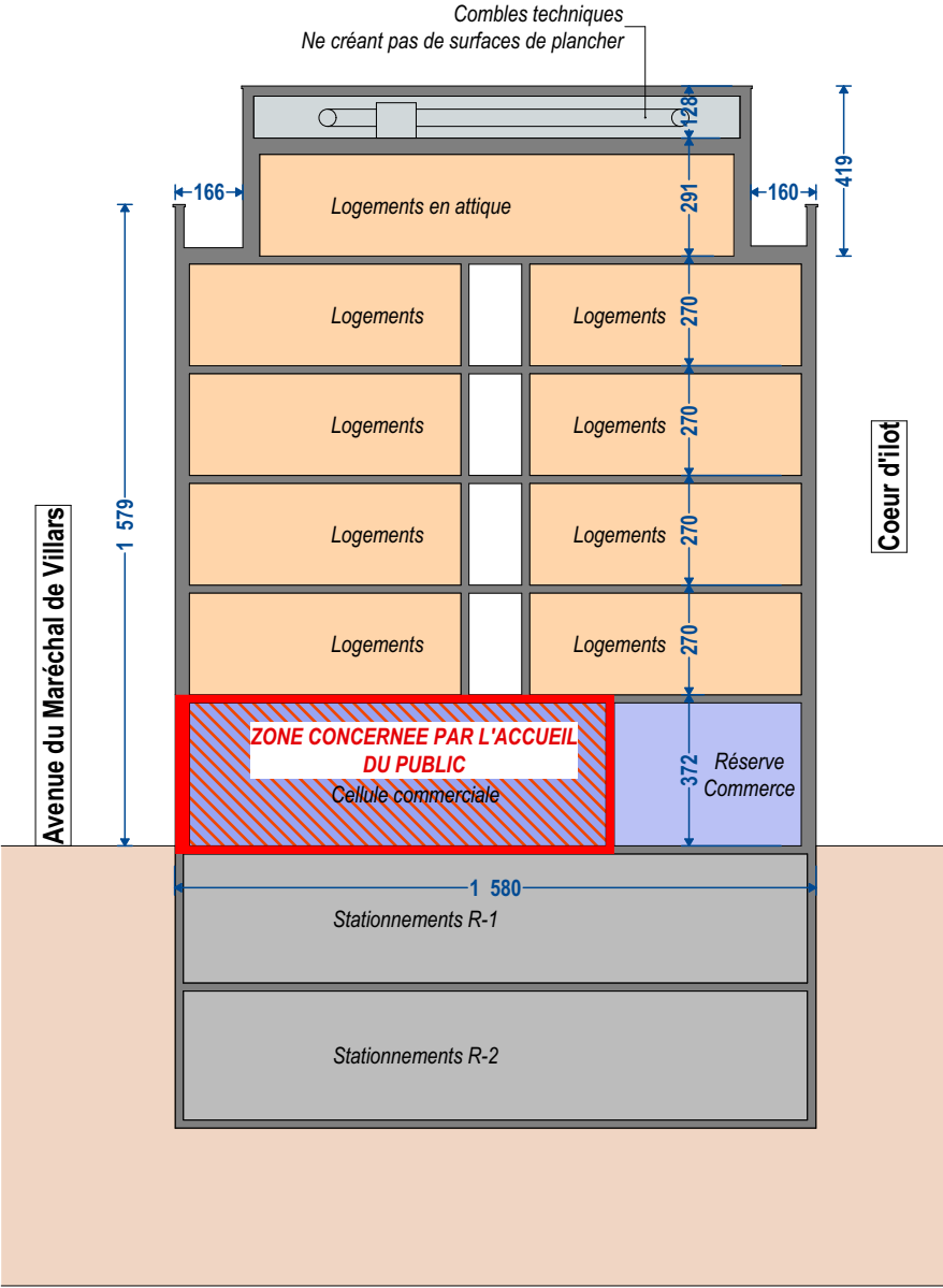
COUPE 1
