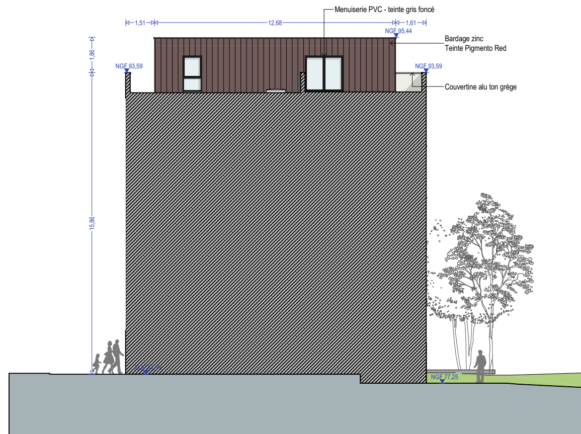
FB-O3 - Façade Ouest #3 (Façade non concernée par l'accueil du public)
