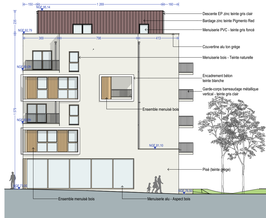
FA1-O1 - Façade Ouest #1
