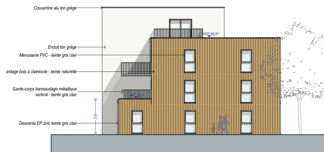
H-02 - Façade Est
