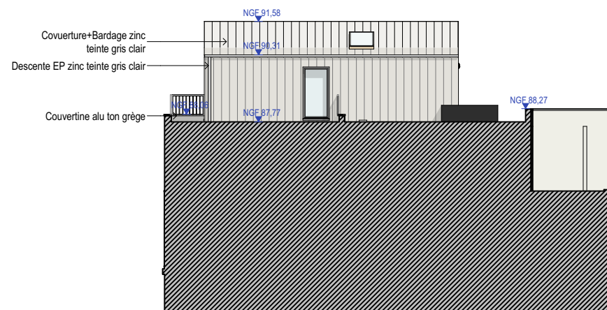
F1-P1 - Pignon 1
