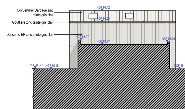
F1-P2 - Pignon 2
