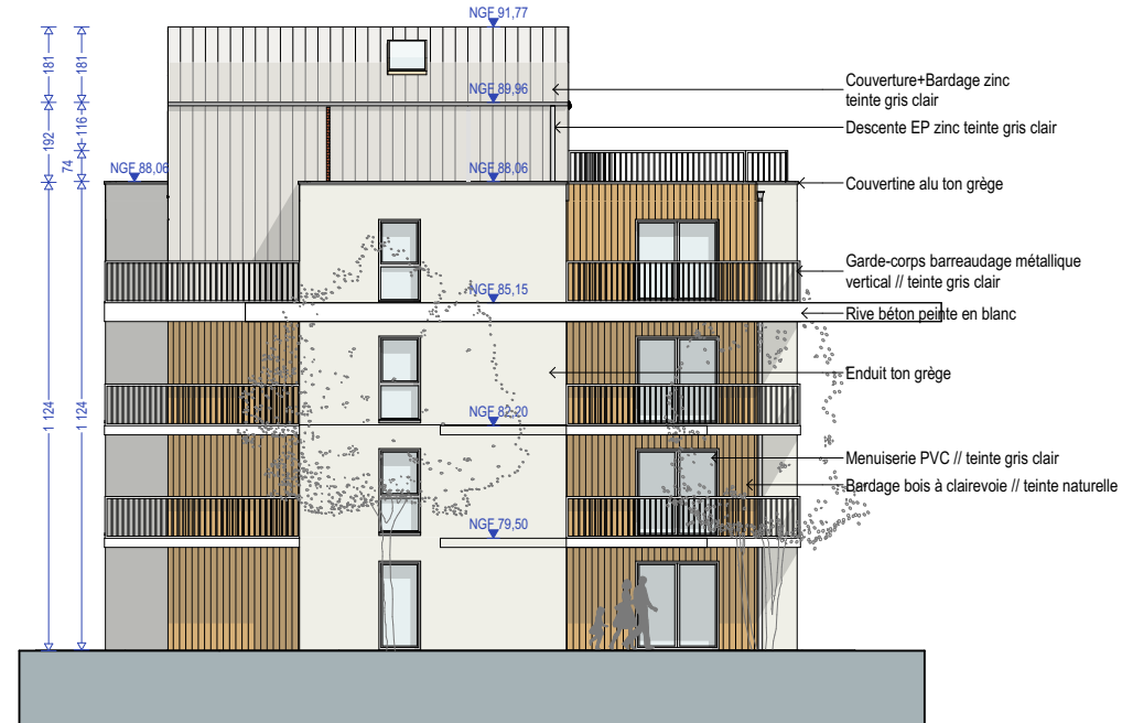
F2-S - Façade Sud depuis venelle
